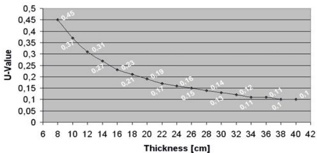
Thermofloc - U-Value
